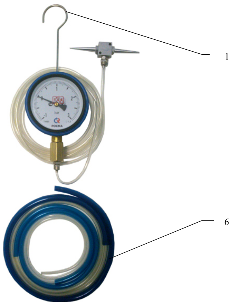
Рис.3 (манометр с трубками)
